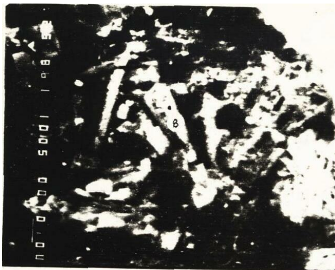
13-расм. Қизилтепа сув қудуқларида ҳосил бўлган чўкманинг арагонит карбонатли кристаллари. (Электрон микроскопда 1290 x катталаштирилган).
